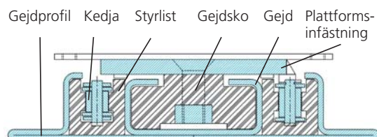
Överföringsenhet med gejd, gejdsko, plattformsinfästning, kedja och styrlist.
